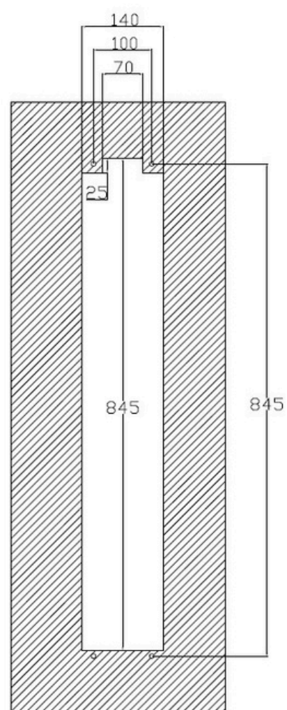
Wymiary otworu montażowego IRGLASSPA
